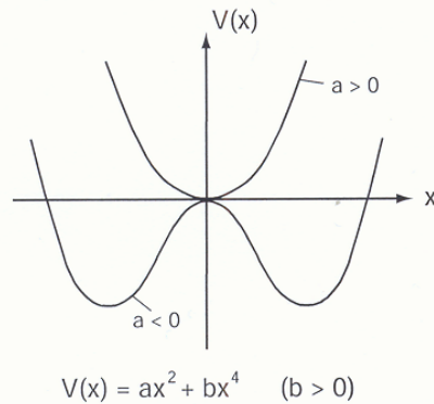
Abb. 3: Deformation eines Potentials ( a > 0 ), dessen Minimum zu einem lokalen Maximum wird ( a < 0 ), neben dem zwei neue Minima entstehen. Ein Zustand im neuen Potential relaxiert aus der vorher stabilen Lösung bei x = 0 in eine der beiden neuen stabilen Lösungen. Da nur je eine dieser beiden Lösungen eingenommen werden kann, spricht man von einem Symmetriebruch.
