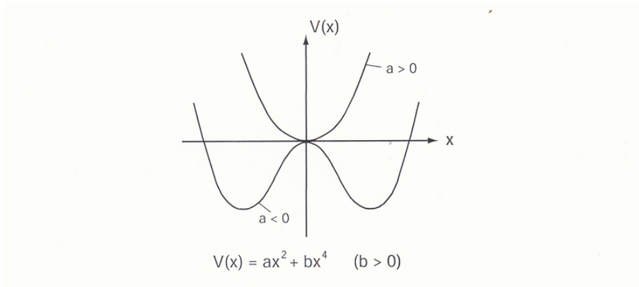
Abb. 6 Deformation eines Potentials ( a > 0 ), dessen Minimum zu einem lokalen Maximum wird ( a < 0 ), neben dem zwei neue Minima entstehen. Ein Zustand im neuen Potential relaxiert aus der vorher stabilen Lösung bei x = 0 in eine der beiden neuen stabilen Lösungen. Da nur je eine dieser beiden Lösungen eingenommen werden kann, spricht man von einem Symmetriebruch.
